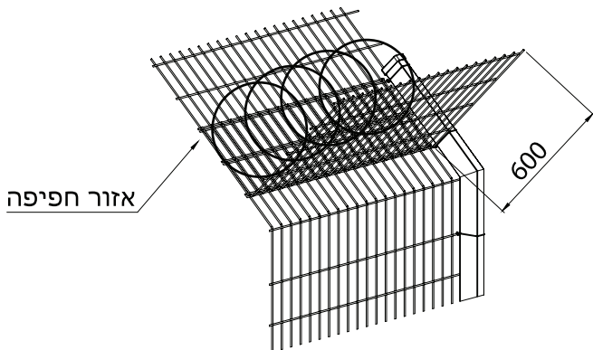
תלתלית ע"ג קרון כפולה
